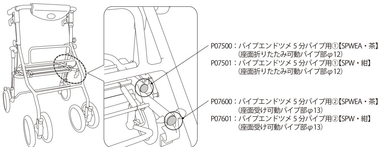
図：シンフォニープラスフレーム全体図
